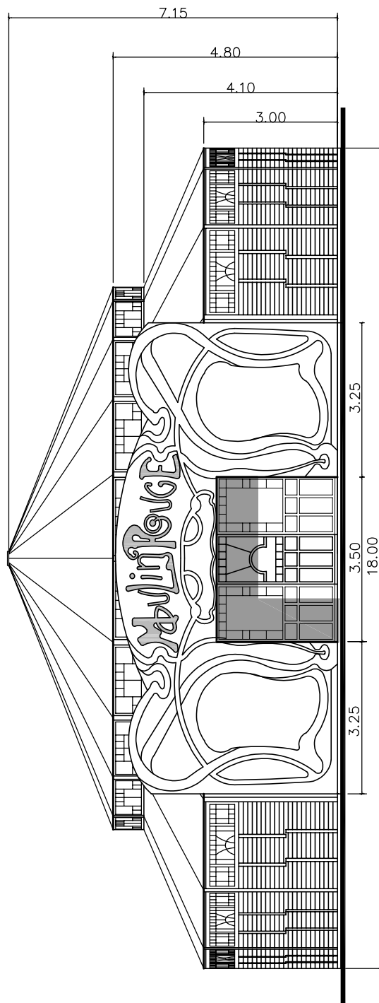
vooraanzicht MOULIN ROUGE
